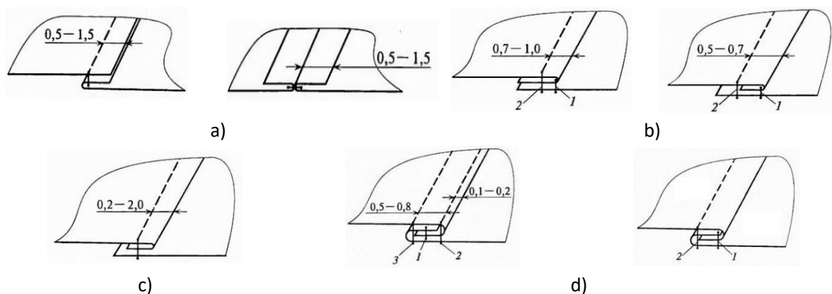
Figura 5.15. Metode de asamblare a corseletelor cu reperele de bază
